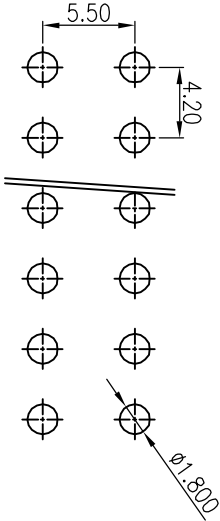
P.C.B LAYOUT
