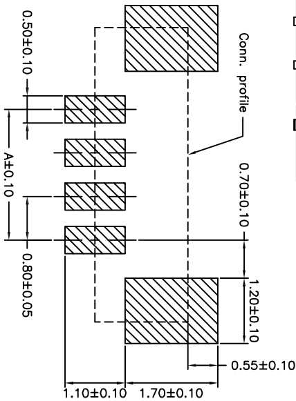
P.C.B. LAYOUT
